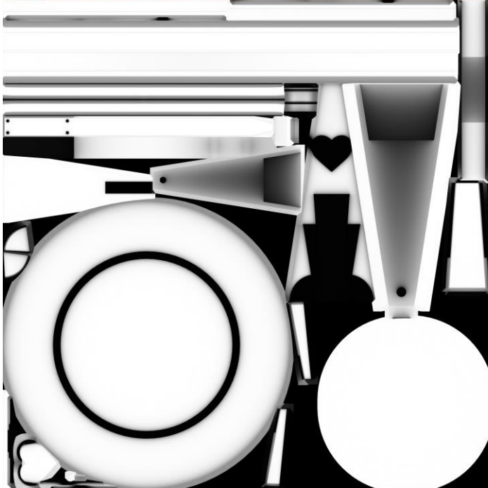
Ambient Occlusion
